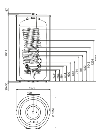
NIBE VPB 1000
