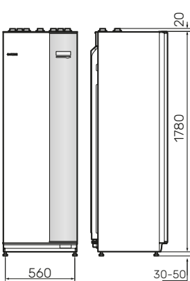
NIBE VVM 310
