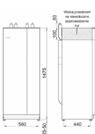
NIBE VPB 200
