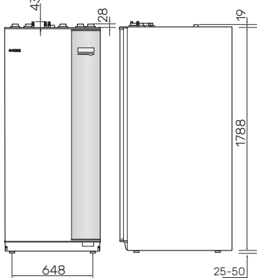
NIBE VVM 500
