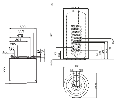
NIBE VPB 500
