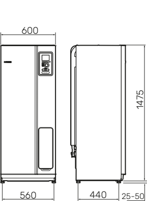
NIBE VVM 225
