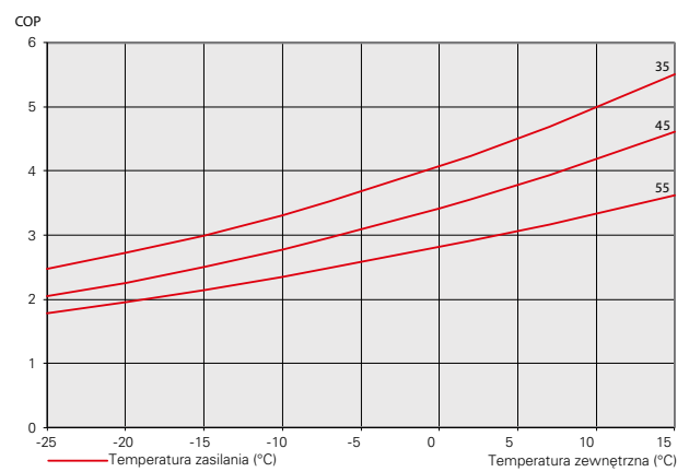
F2120-20 COP
