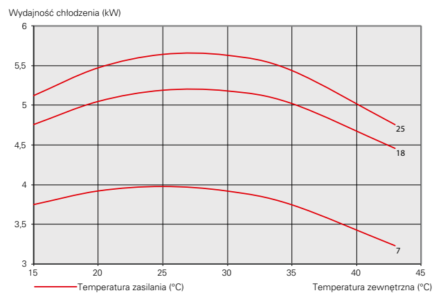
F2120-8
