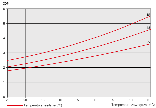
F2120-16 COP
