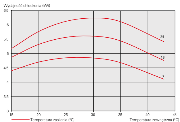
F2120-16
