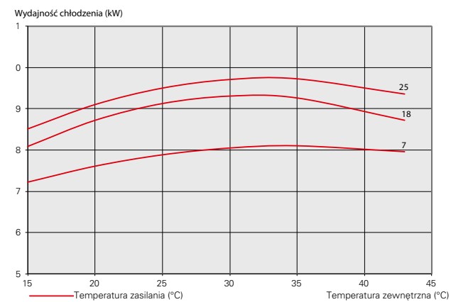
F2120-20
