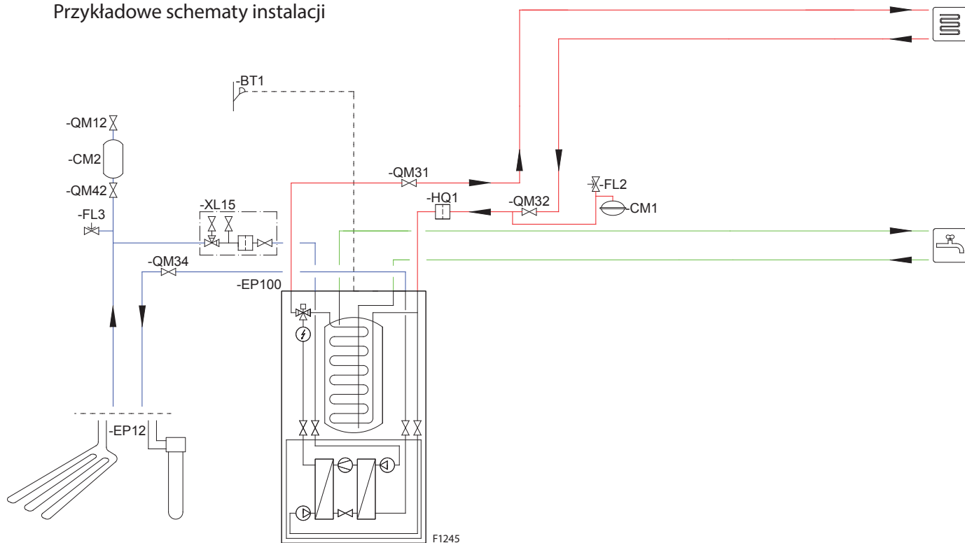
Schemat F1245 z jednym obiegiem grzewczym
