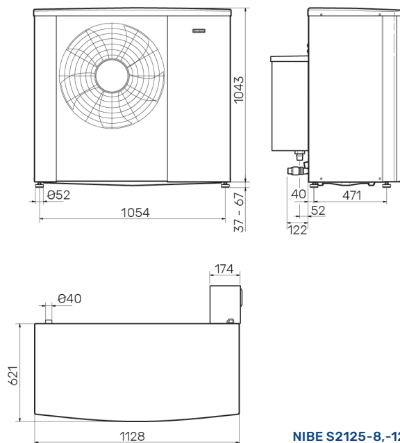
NIBE S2125-8,-12
