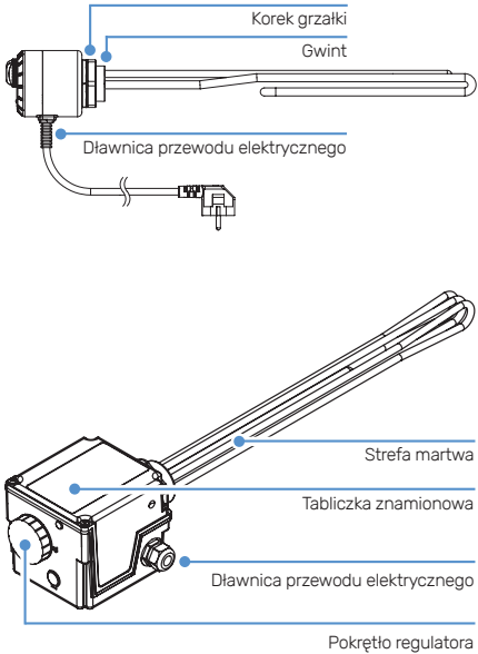
Budowa elektrycznych modułów grzejących ME-0040 - ME 2120
