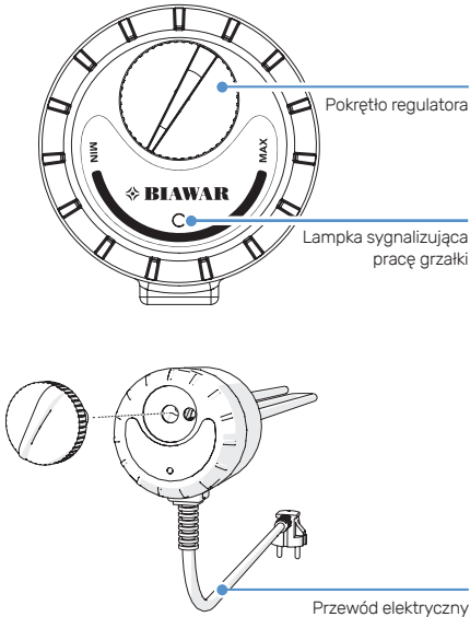
Budowa elektrycznych modułów grzejących ME 0015 - ME 0030
