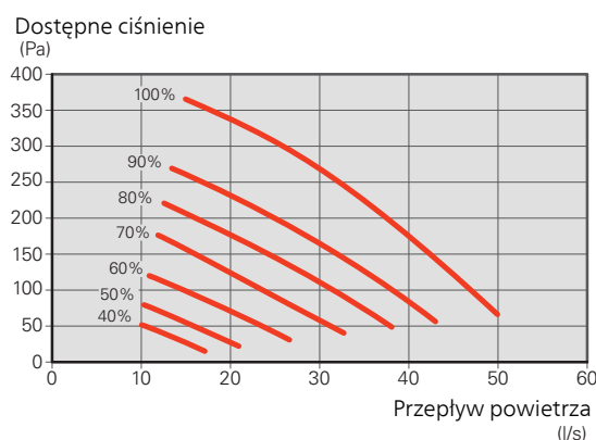
Wydajność wentylacji GV-HR 130-250
