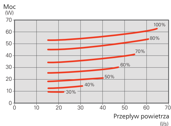
Moc wentylatora 1 GV-HR 130-250
