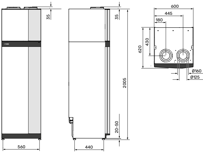
NIBE S735
