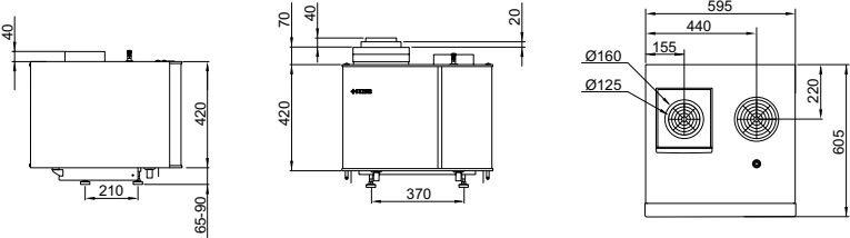
NIBE F130
