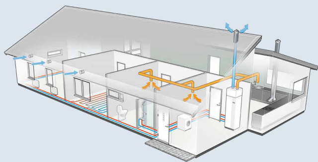
NIBE F370
