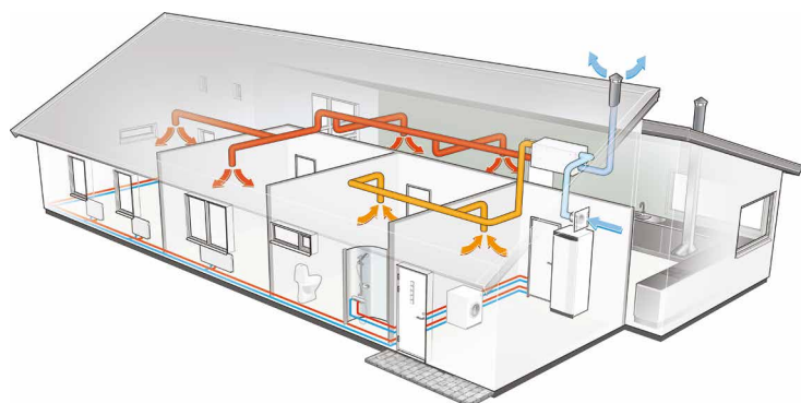
NIBE ERS 30-550
