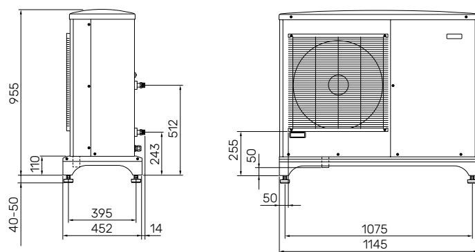
NIBE F2040-12
