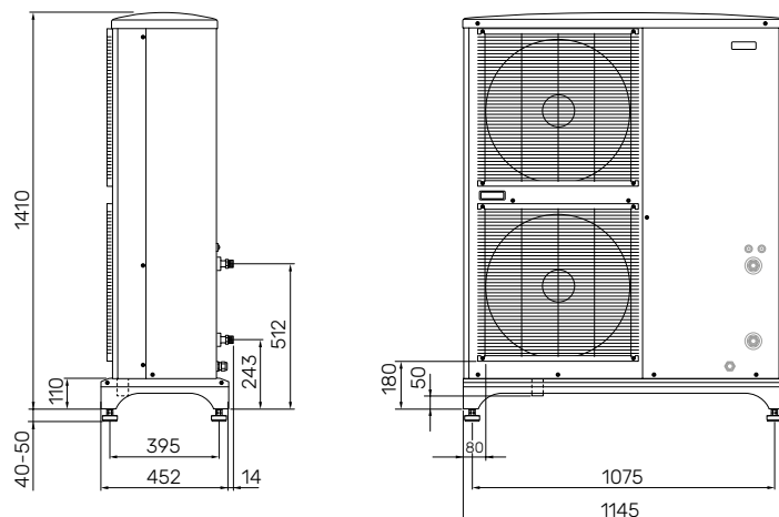
NIBE F2040-16
