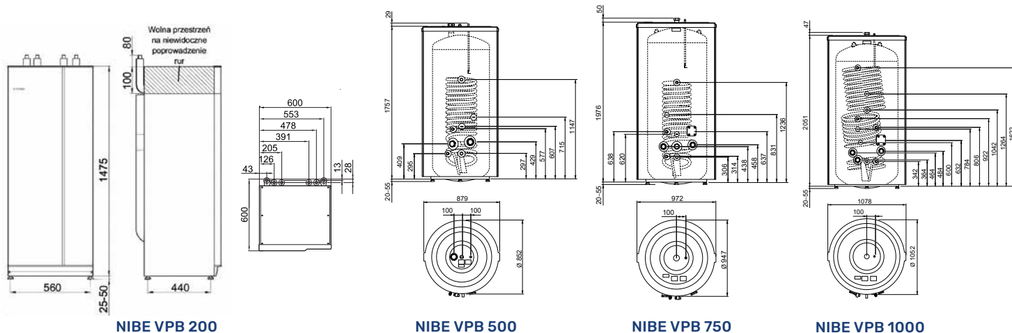
NIBE VPB 200
